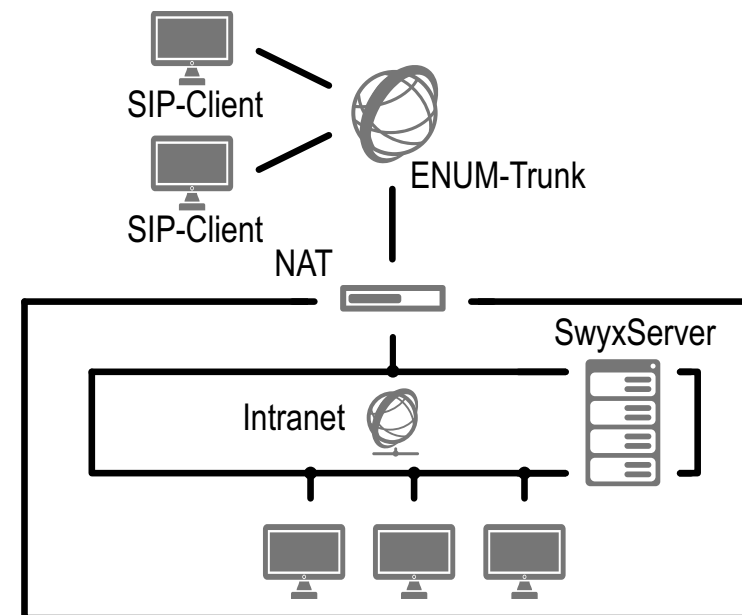
Abb. 18-1: SIP ohne Internet Service Provider (ITSP)
