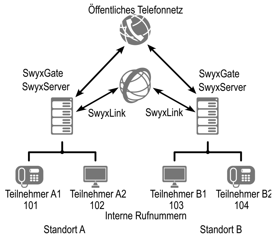
Abb. 17-1: Standortkopplung als Server-Server-Kopplung
