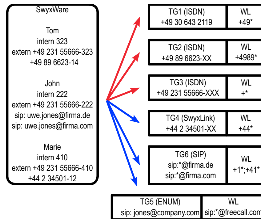
Abb. 10-1: Beispielkonfiguration für einen Rufnummernplan, Trunk-Gruppen (TG) und Weiterleitungen (WL)
