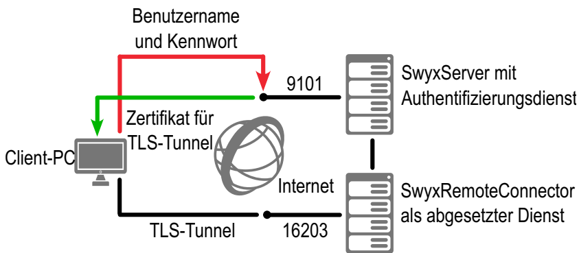
Abb. 26-1: Verbindungsaufbau via Authentifizierungsdienst
