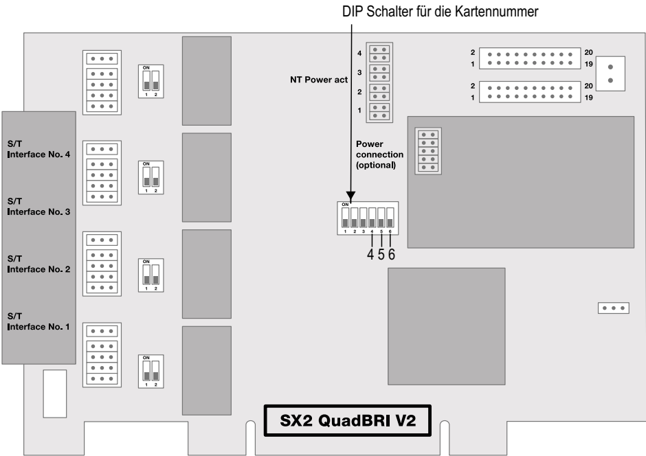
Abb. 15-1: Kartennummer-Konfiguration der SX2-express QuadBRI
