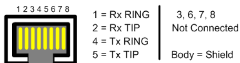
Abb. C-6: RJ-48c Pinbelegung eines E1/T1 PRI-Einschubmoduls
