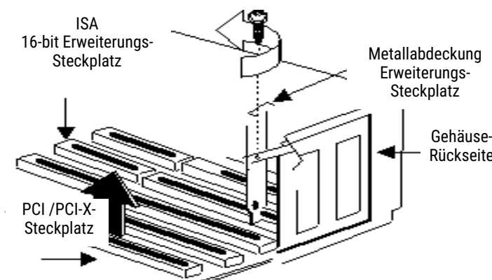
Abb. 15-5: Entfernen der Metallabdeckung
