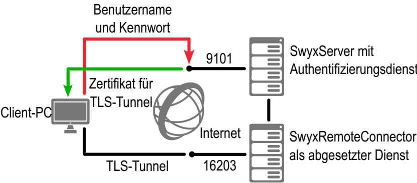
Abb. 26-2: Verbindungsaufbau via Authentifizierungsdienst
