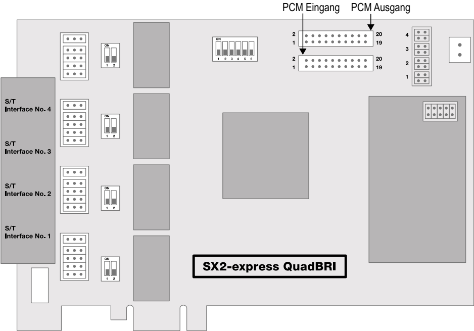
Abb. 15-2: PCM-Verbindung der SX2-express QuadBRI
