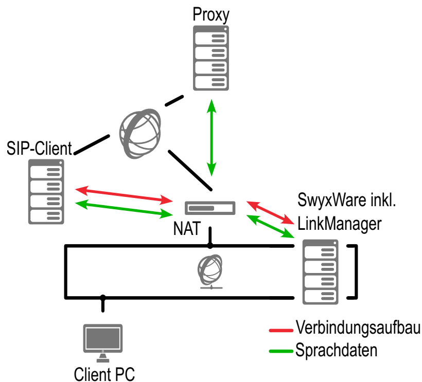
Abb. 16-1: Szenario - Gespräche über SIP
