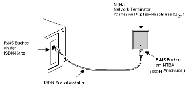
Abb. 15-6: Anschluss des ISDN-Kabels
