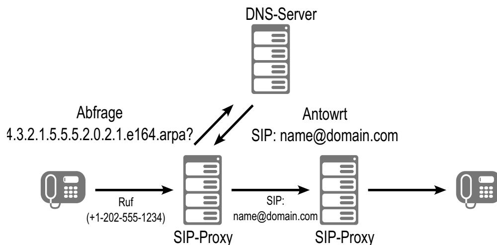
Abb. 18-2: ENUM-Anrufprozess
